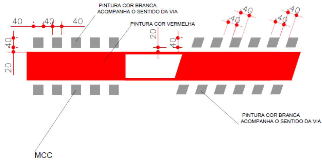
DETALHE CRUZAMENTO RODOCICLOVIÁRIO
