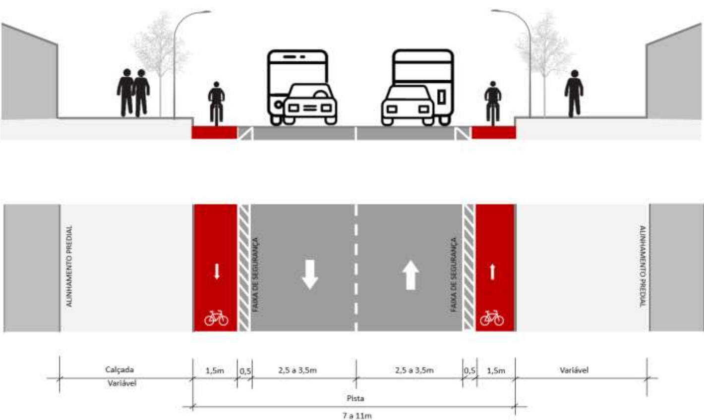
P4 - PADRÃO CICLOFAIXA 1,5M + 0,5 FAIXA DE SEGURANÇA
