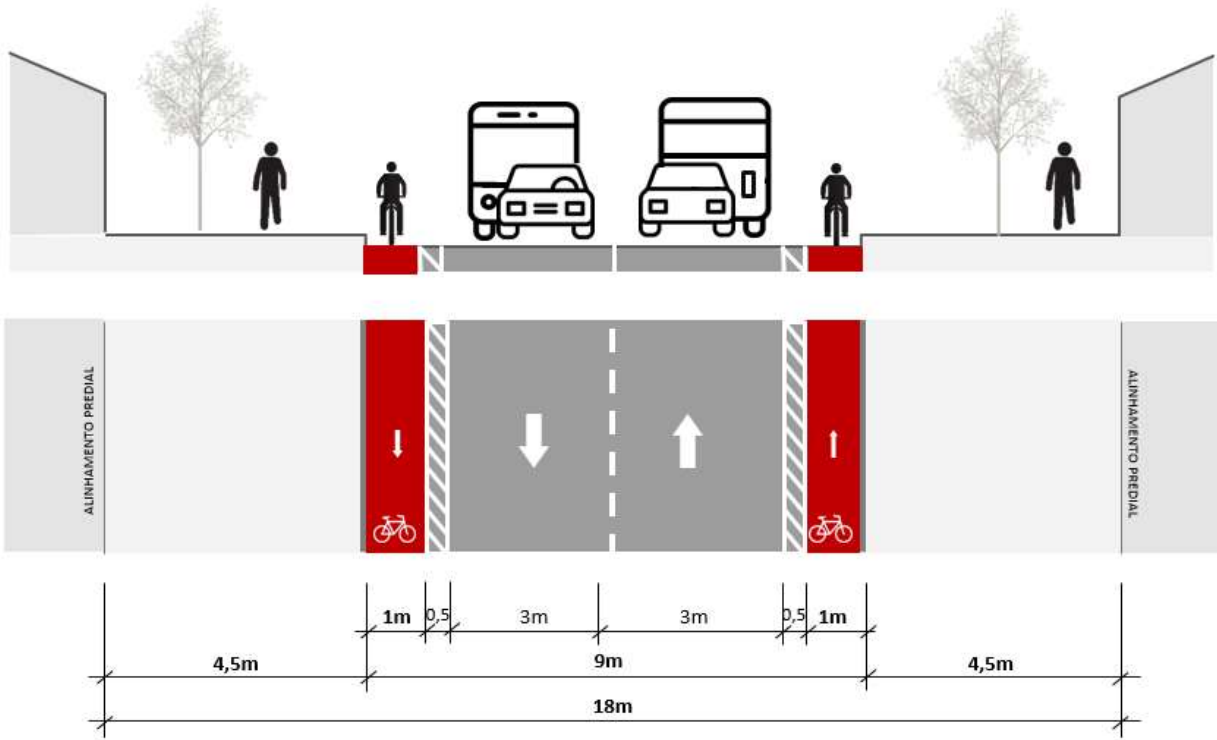
P3 sem estacionamento sentido duplo
