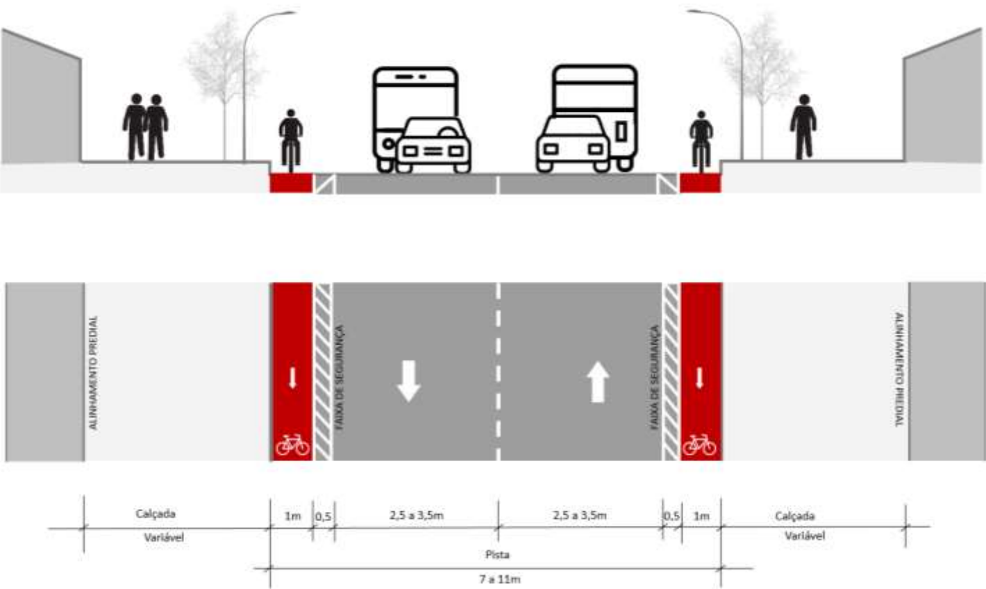
P3 - PADRÃO CICLOFAIXA 1M + 0,5 FAIXA DE SEGURANÇA
