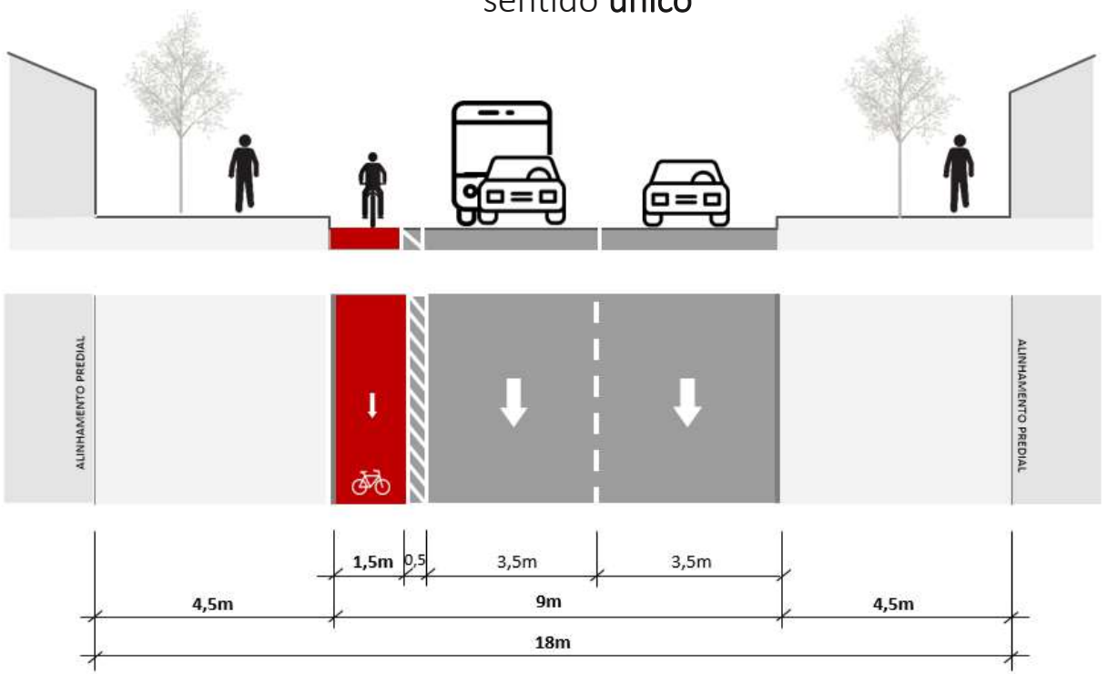
P4 sem estacionamento sentido único
