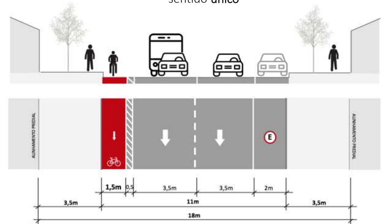
P4 1 estacionamento sentido único
