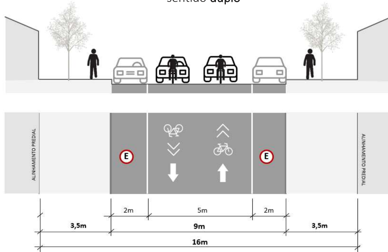
P1 2 estacionamentos sentido duplo
