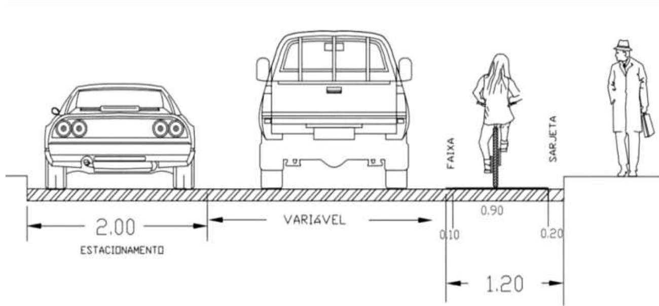
DETALHE PERFIL TIPO - VIA LENTA
