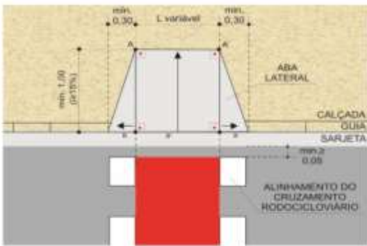
DETALHE REBAIXAMENTO DE CALÇADA RODOCICLOVIÁRIO
