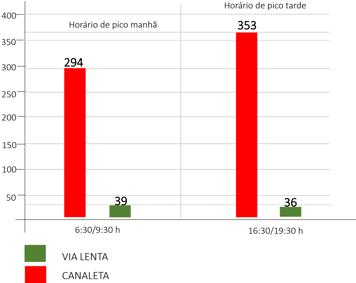
Contagem de tráfego de Bicicletas horário de pico - Canaleta/ Via Lenta Avenida República Argentina – Trecho 2 Av. Arthur Bernardes/Rua Carlos Dietzsch
