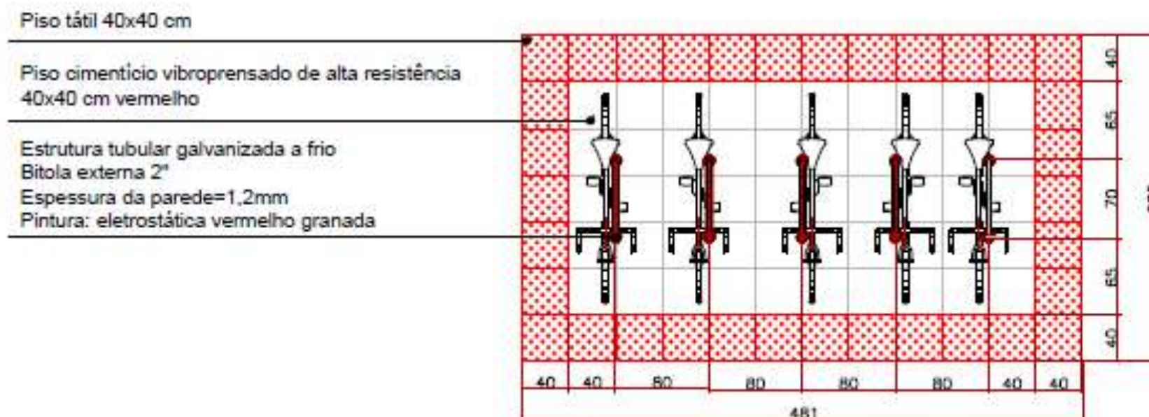
PLANTA ESC. 1:50
