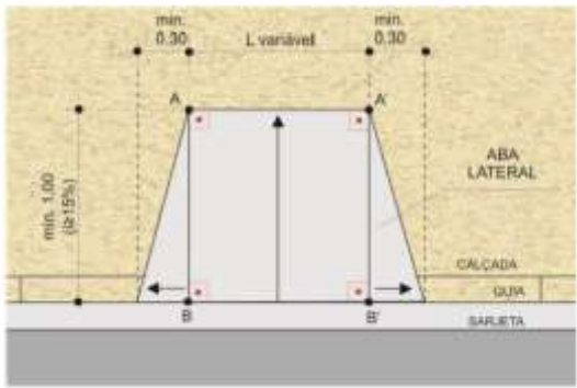
DETALHE REBAIXAMENTO DE CALÇADA
