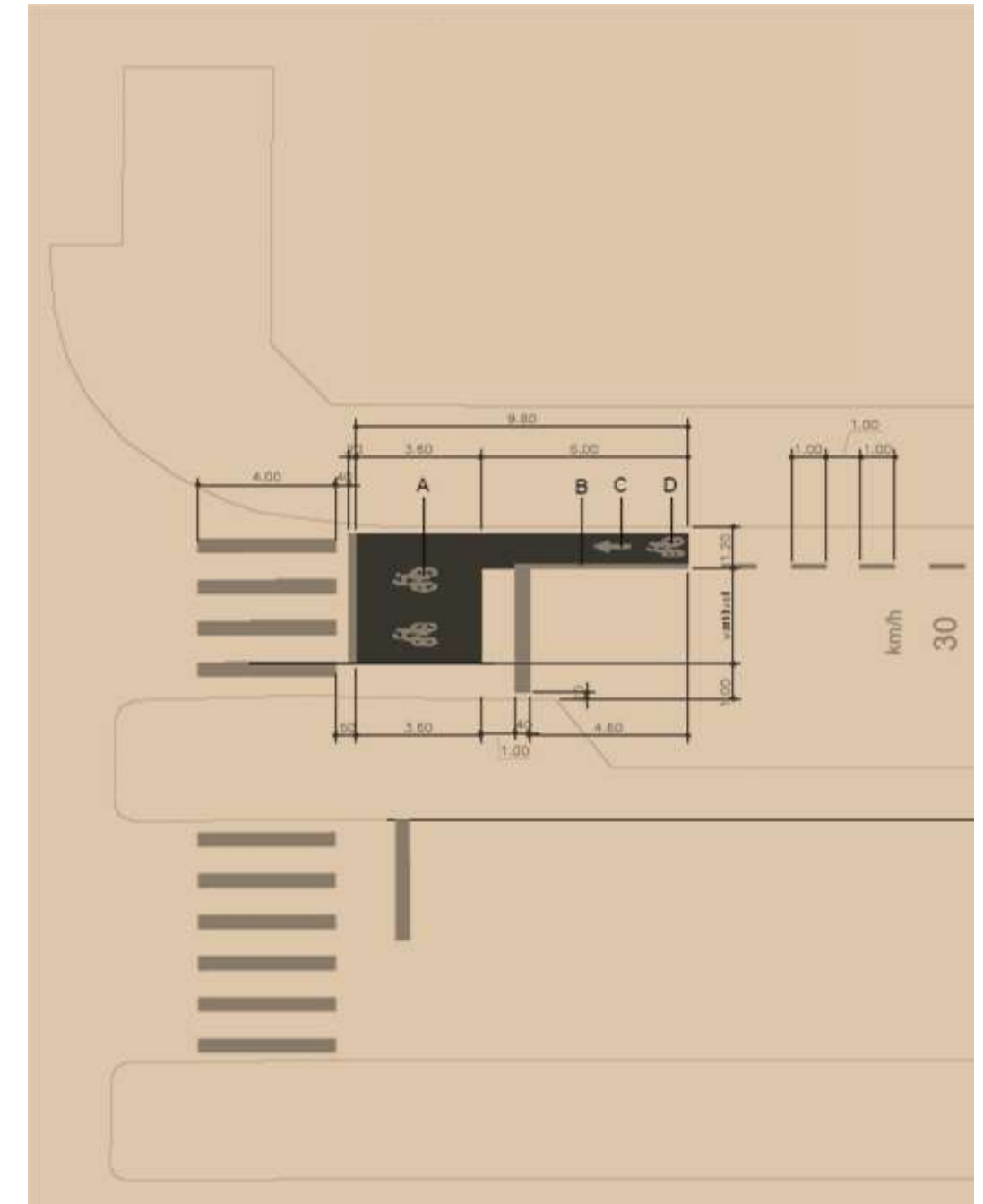
DETALHE BICICAIXA VIA LENTA - SE
