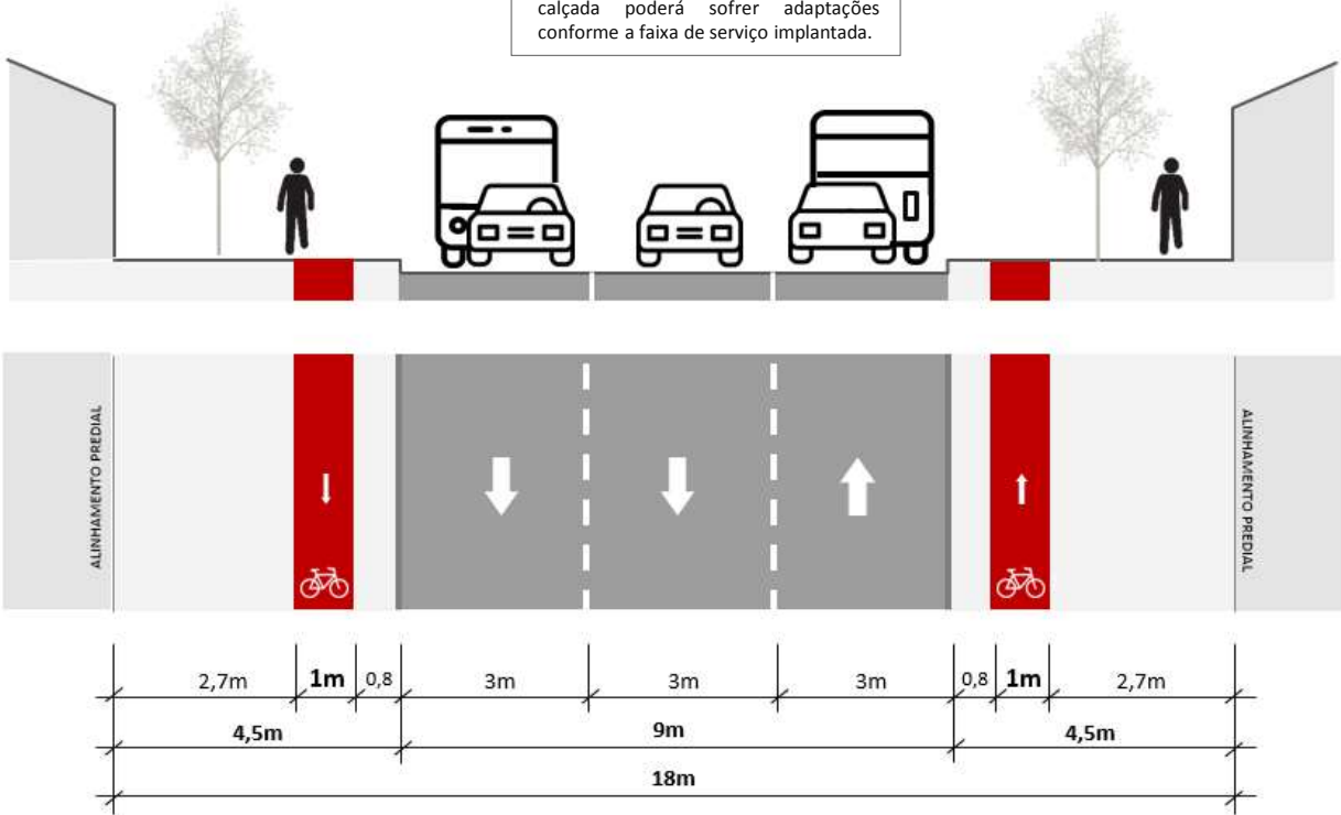
P2 sem estacionamento sentido duplo
