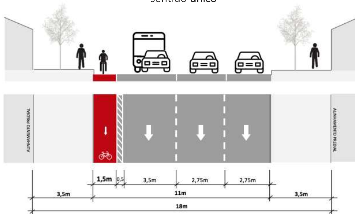
P4 sem estacionamento sentido único
