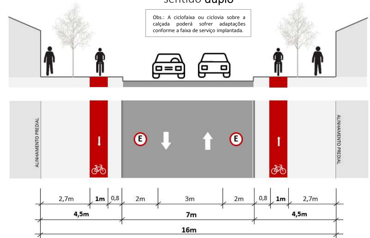
P2 2 estacionamentos sentido duplo
