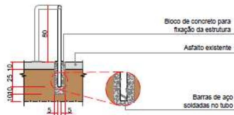
CORTE TRANSVERSAL ESC.: 1:25
