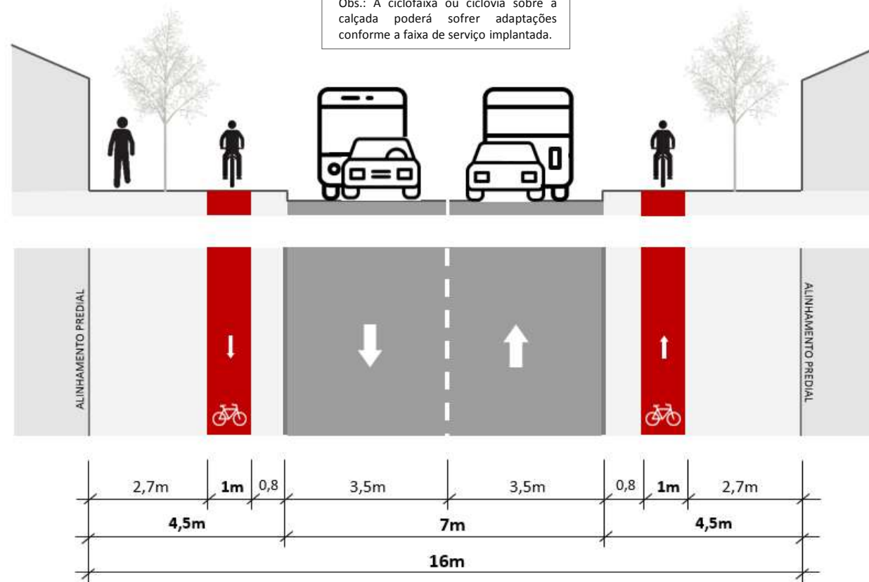
P2 sem estacionamento sentido duplo
