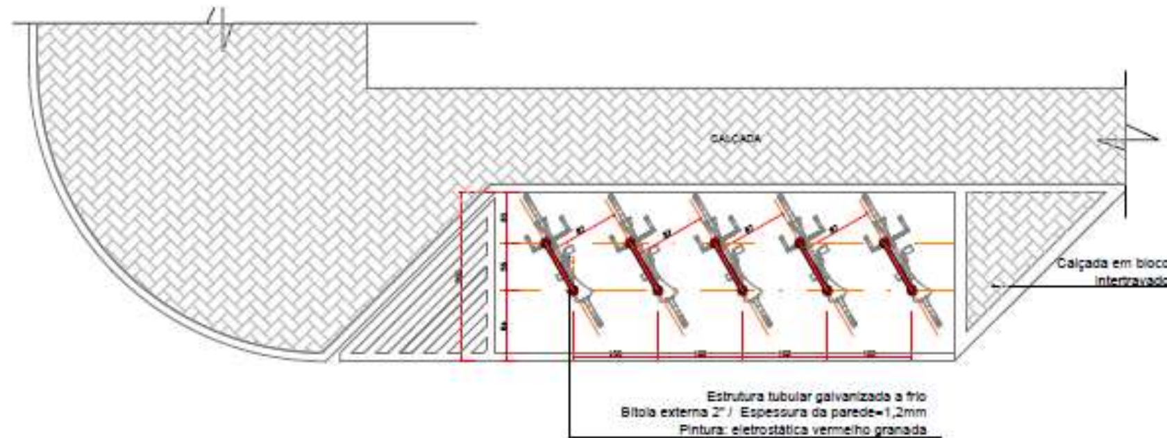
PLANTA ESC.: 1:50
