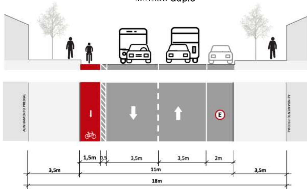
P4 1 estacionamento sentido duplo
