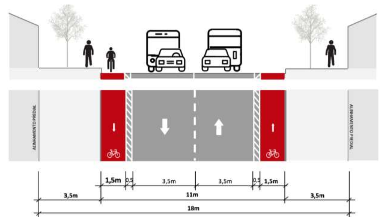
P4 sem estacionamento sentido duplo
